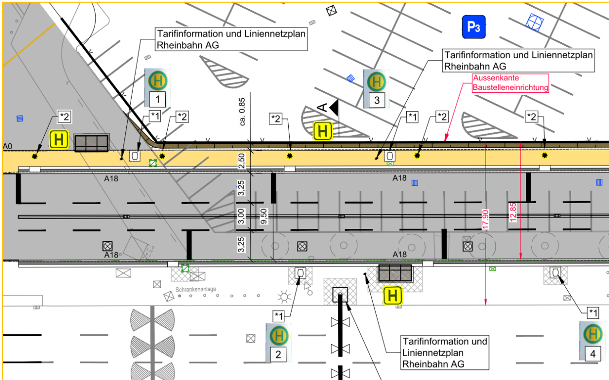
Auszug Lageplan
