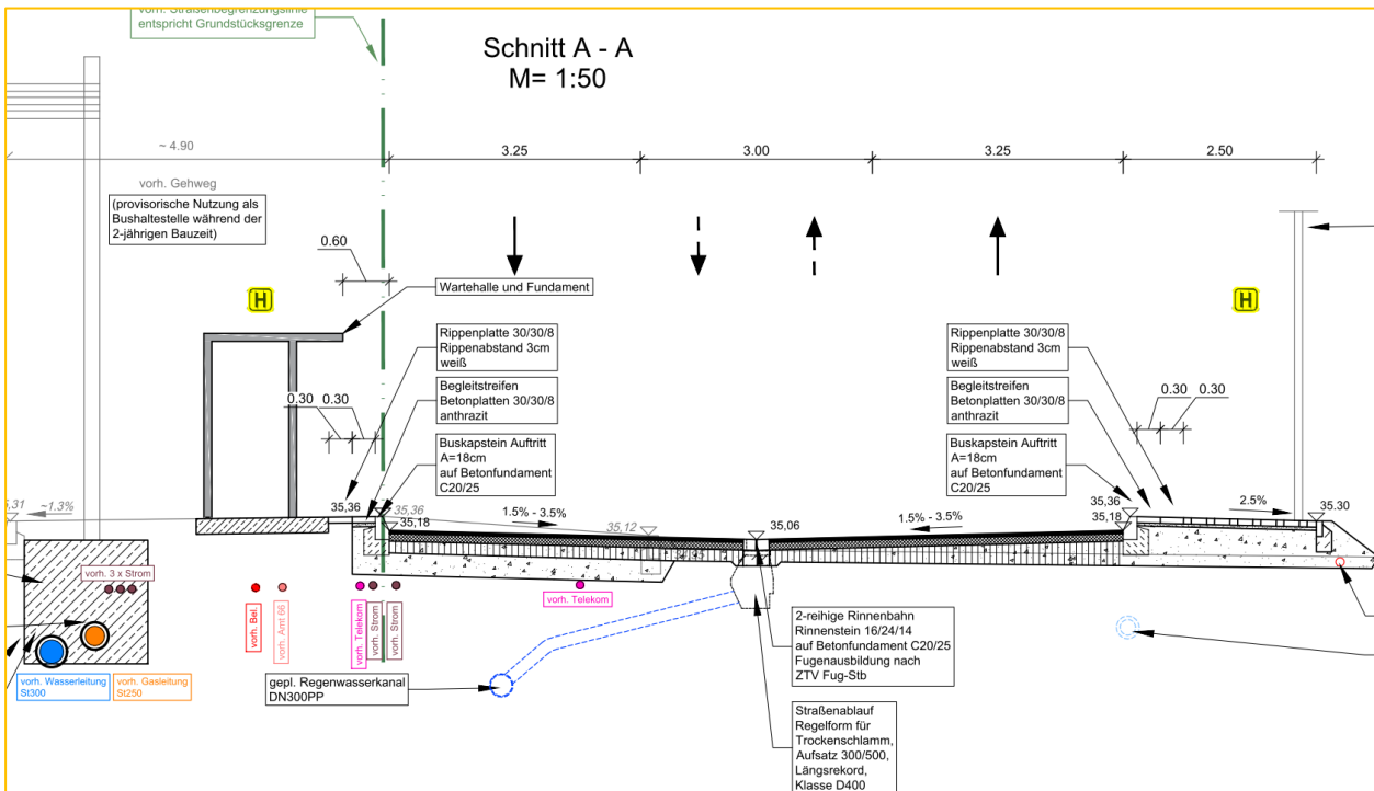
Auszug Ausbauquerschnitt
