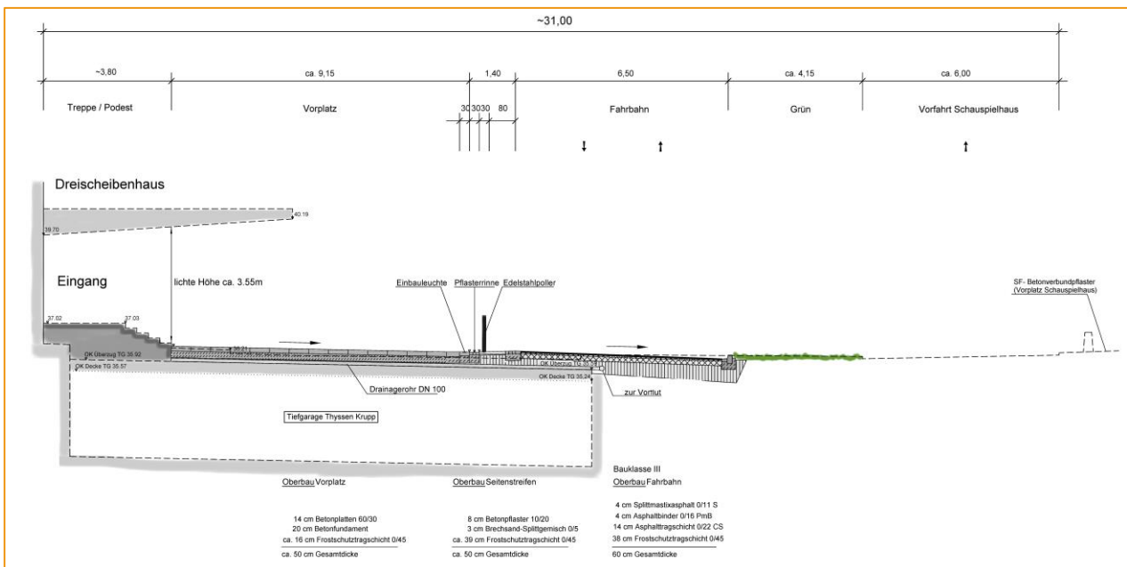
Querschnitt Platzbereich
